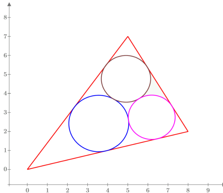
Рис. 10 Графическое отображение решения задачи Мальфатти
