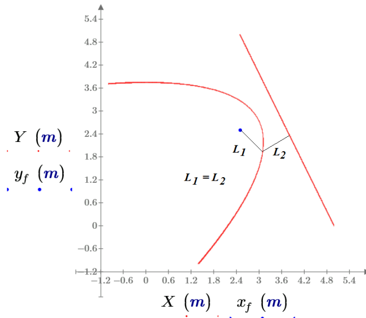
Рис. 12 Построение параболы и ее директрисы сканированием плоской области (примечание: на графике тонкие прямые линии и буквенные обозначения дорисованы в ручном режиме)
