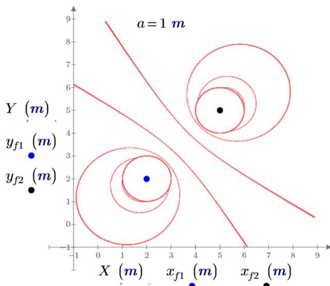
Рис. 14 Построение семейства окружностей Аполлония
