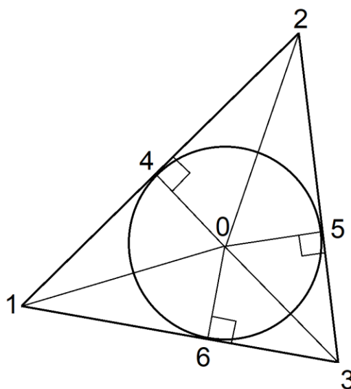
Рис. 1. Схема задачи об окружности, вписанной в треугольник
