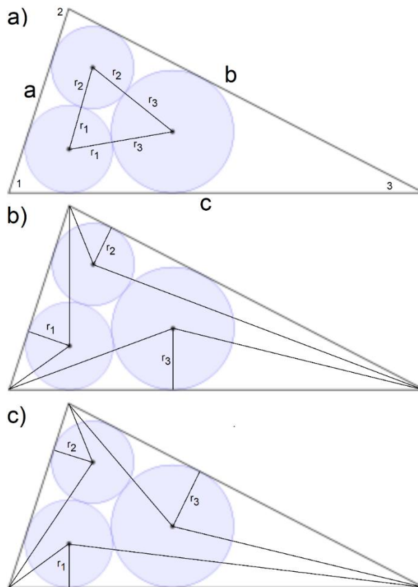
Рис. 8 Три схемы задачи об окружностях Мальфатти
