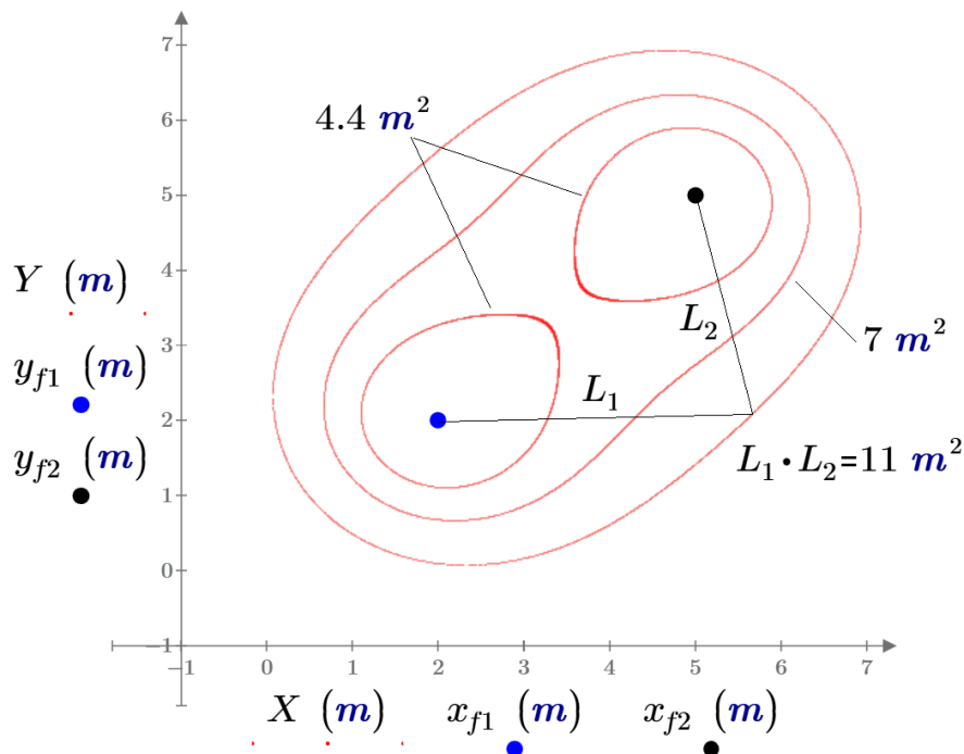
Рис. 13 Построение овалов Кассини сканированием области (примечание: на графике тонкие прямые линии-указатели и буквенные обозначения дорисованы в ручном режиме)
