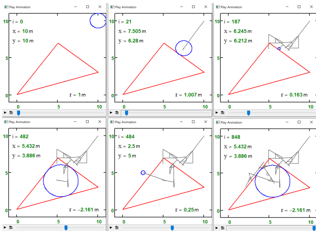
Рис. 11 Трассировка численного решения задачи об окружности, вписанной в треугольник
