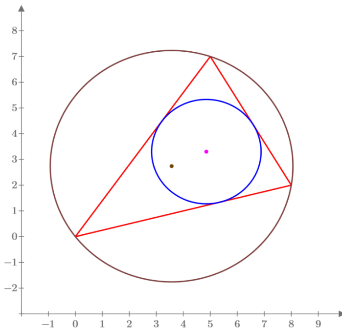
Рис. 5 Треугольник с вписанной и описанной окружностями
